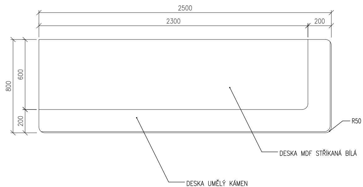
PŮDORYS 1:20
