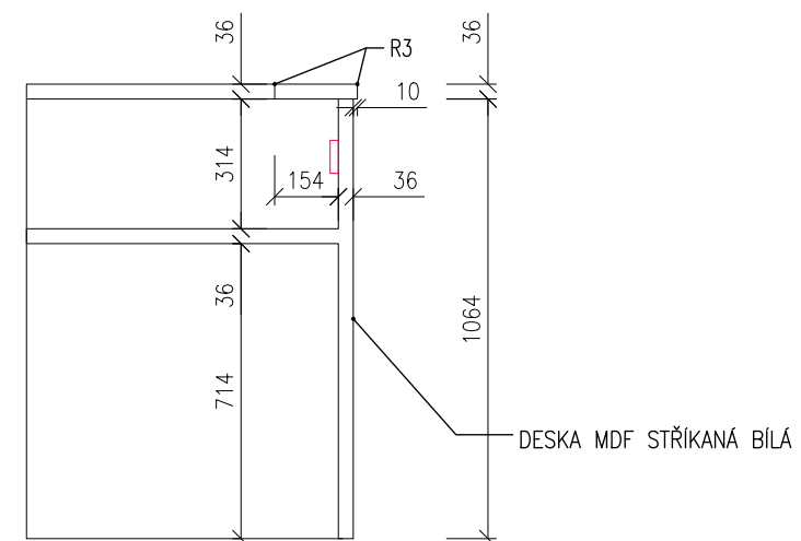
ŘEZ 1:20
