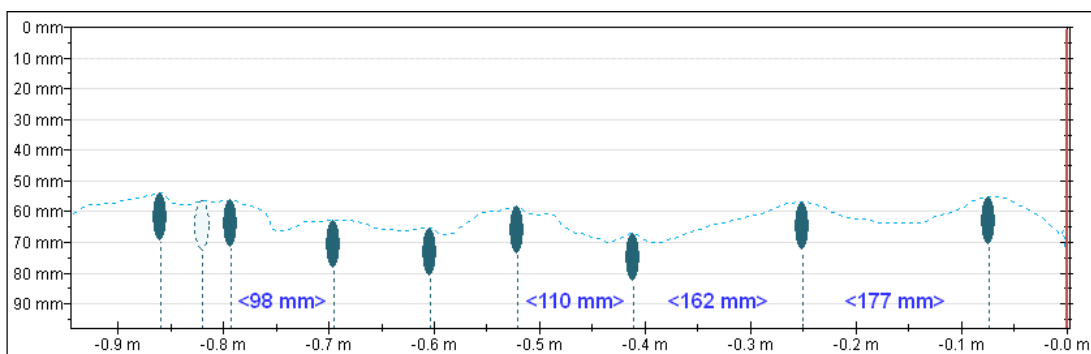
Obr. č. 32: výstup z přístroje – poloha výztuže, červená čára vpravo značí začátek měření pod stropem
